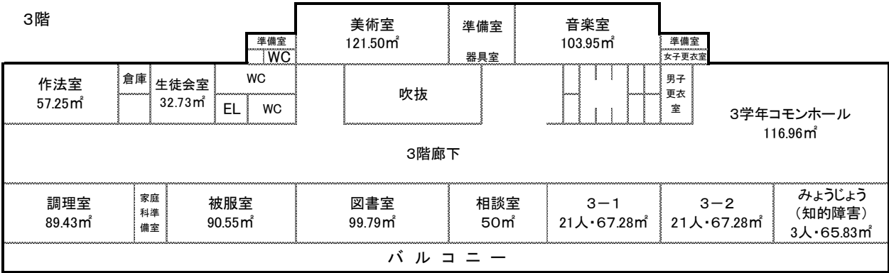
津谷中学校校舎各階平面図
